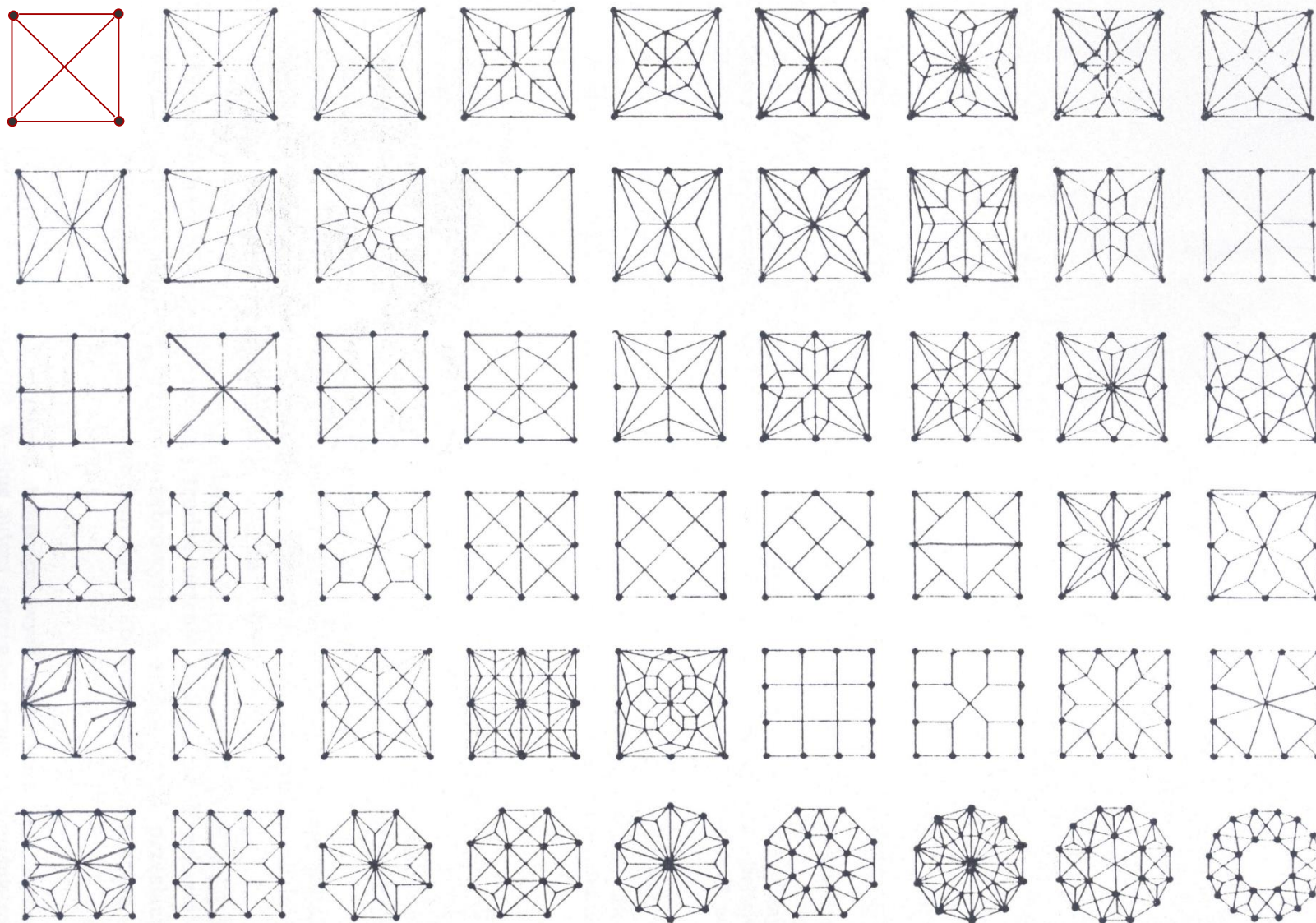
Rys. 5—20. Wzory geometryczne rzutu sklepień gotyckich w zależności od punktów podparcia i powierzchni sklepiennego pola
